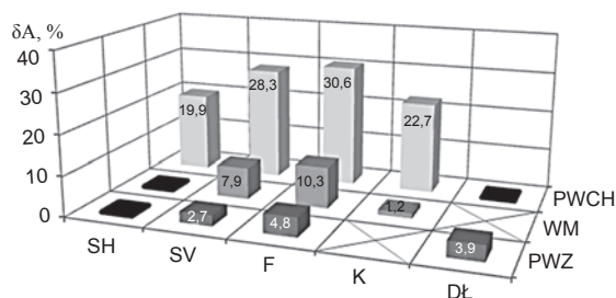
Rys. 12. Porównanie względnych oszczędności energii przy zastosowaniu różnych rodzajów regulacji dla rozpatrywanych urządzeń (czarne prostokąty to warianty najmniej korzystne dla danego urządzenia)
