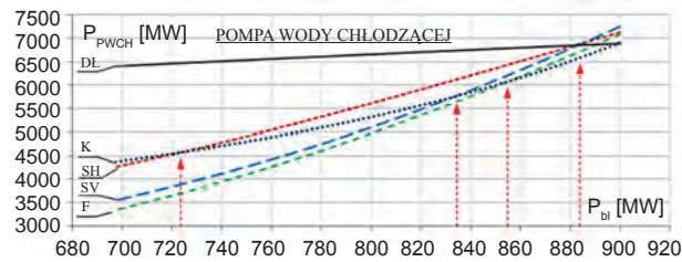
Rys. 7. Porównanie zmienności obciążeń elektrycznych dla różnych układów napędowych pompy wody chłodzącej, wentylatora młynowego SV – sprzęgło Vorecon, SH – sprzęgło standardowe, F – falownik, DŁ – dławienie, K – kierownice na wlocie
