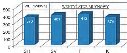
Rys. 11. Porównanie rocznych wskaźników efektywności energetycznej dla różnych wariantów regulacji wentylatora młynowego
