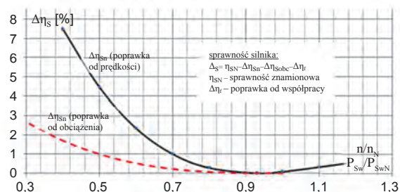
Rys. 4. Sprawność silnika elektrycznego w zależności od względnego obciążenia na wale i względnej prędkości obrotowej
