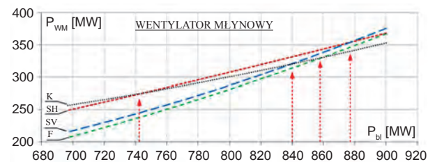
Rys. 8. Porównanie zmienności obciążeń elektrycznych dla różnych układów napędowych wentylatora młynowego SV – sprzęgło Vorecon, SH – sprzęgło standardowe, F – falownik, DŁ – dławienie, K – kierownice na wlocie
