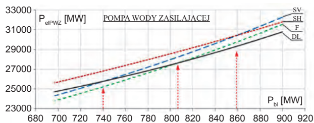
Rys. 6. Porównanie zmienności obciążeń elektrycznych dla różnych układów napędowych pompy wody zasilającej SV – sprzęgło Vorecon, SH – sprzęgło standardowe, F – falownik, DŁ – dławienie, K – kierownice na wlocie
