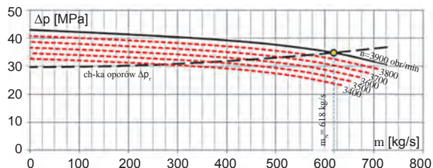
Rys. 2. Charakterystyki przepływowe pompy wody zasilającej dla różnych prędkości obrotowych wirnika oraz charakterystyka oporów układu (rurociągu)
