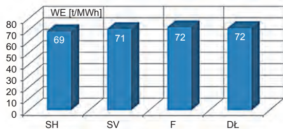
Rys. 9. Porównanie rocznych wskaźników efektywności energetycznej dla różnych wariantów regulacji pompy zasilającej
