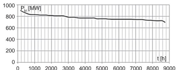
Rys. 1. Uporządkowany wykres obciążeń bloku energetycznego przyjęty do obliczeń
