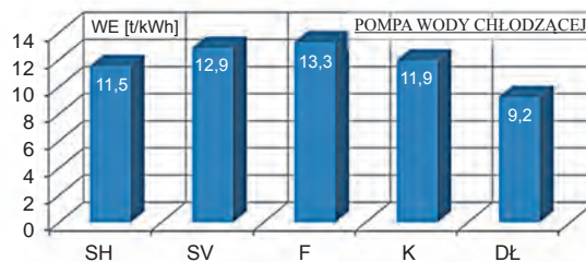
Rys. 10. Porównanie rocznych wskaźników efektywności energetycznej dla różnych wariantów regulacji pompy chłodzącej
