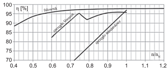
Rys. 5. Sprawności sprzęgieł hydrokinetycznych i falownika w zależności od względnej prędkości obrotowej napędu
