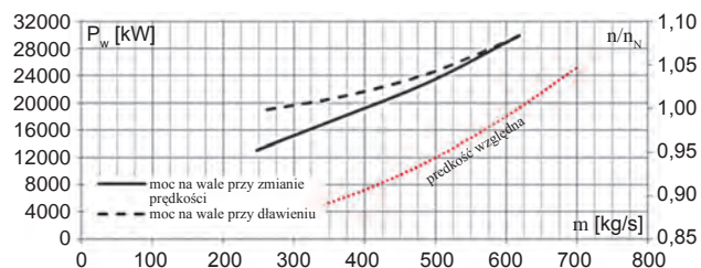
Rys. 3. Zmiana mocy na wale pompy zasilającej oraz charakterystyka regulacyjna przy różnych rodzajach regulacji wydajności
