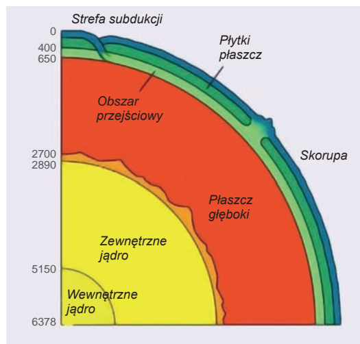
Rys. 1. Budowa wnętrza Ziemi
